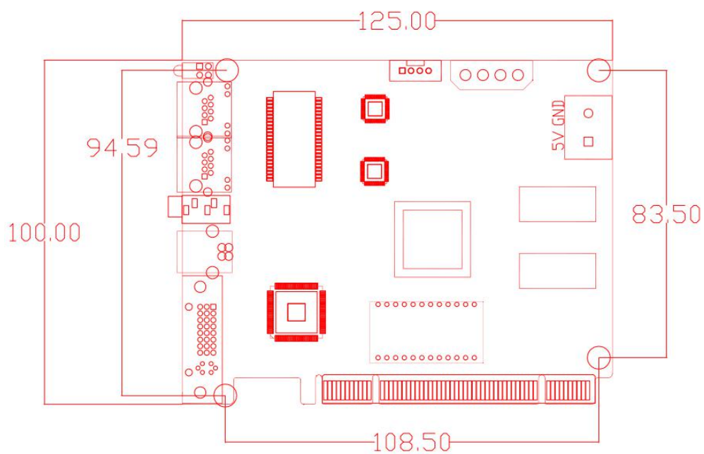
V9 孔位图
