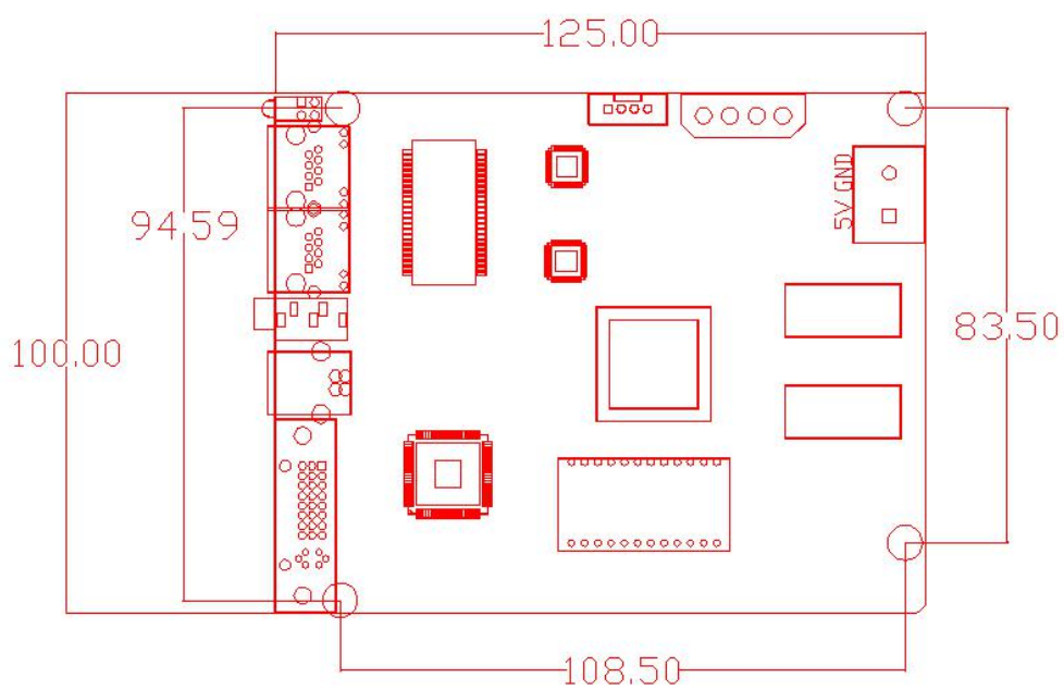
V9BOX 孔位图
